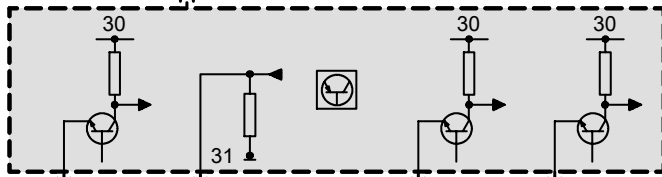
A23 Driver's door module
