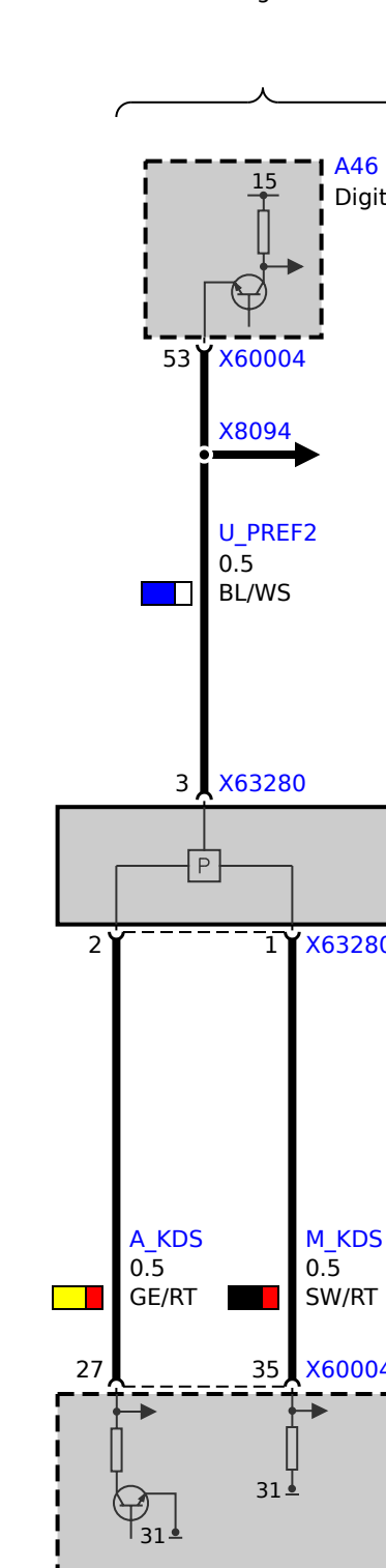
N63 engine
