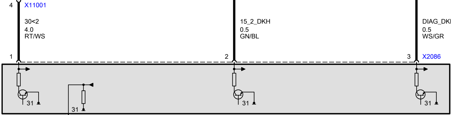
E2000 Fuel heater
